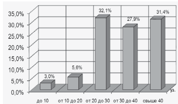
Рис. 3. Применение водометных движителей на кораблях различных стран в зависимости от скорости, уз
