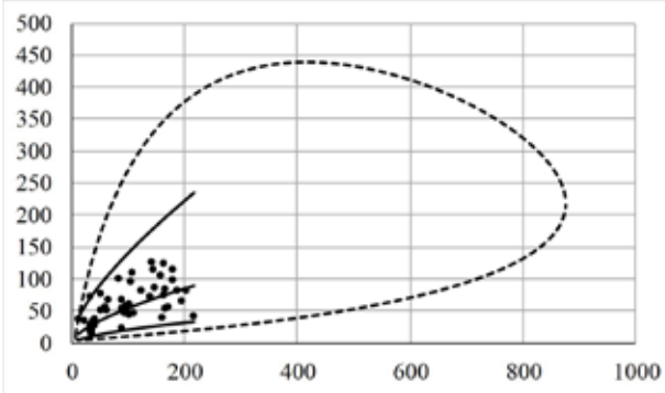
Рис. 3. Нелінійна регресія, побудована з використанням нормалізуючого перетворення на основі десяткового логарифму
