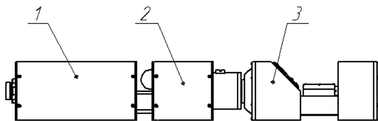
Рисунок 2 – Конструкція прив'язної свердловинної відеокамери.
